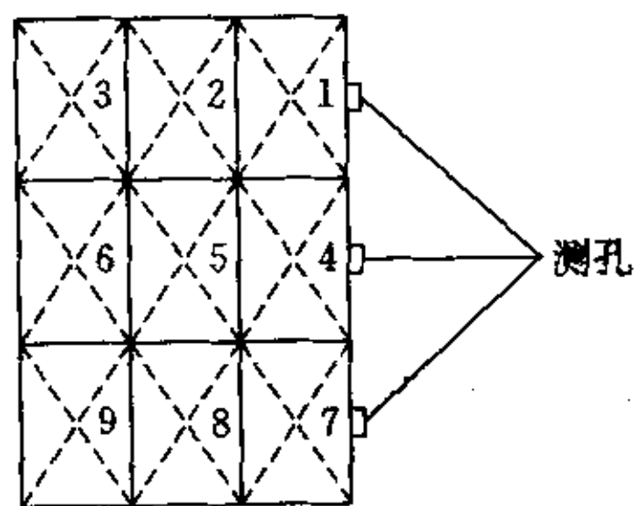
图 2 矩形管道测点位置
